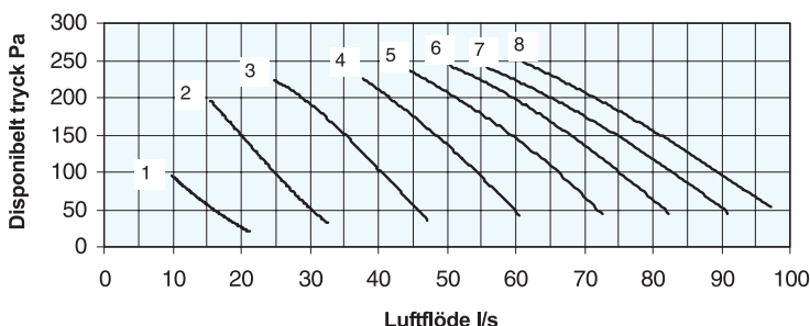
PINGVIN ACE FRÄNLUFT Specifika kurvor med EU5 PLANFILTER 1, 2, 3, 4, 5, 6, 7 och 8 hastighet
