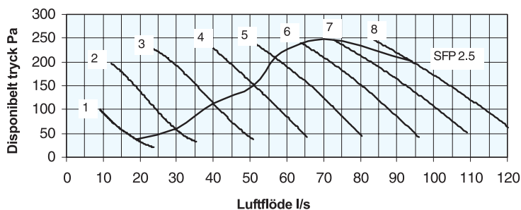
PINGVIN AC och ACW FRÄNLUFT Specifika kurvor med EU5 PLANFILTER 1, 2, 3, 4, 5, 6, 7 och 8 hastighet
