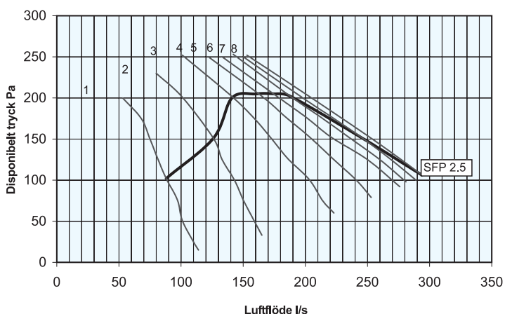
PEGASOS AC, FRÅNLUFT Specifika kurvor med EU4/5 FILTER 1, 2, 3, 4, 5, 6, 7 och 8 hastighet
