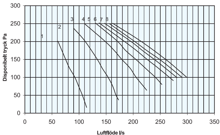
PEGASOS AC, TILLUFT Specifika kurvor med EU 4/5 FILTER 1, 2, 3, 4, 5, 6, 7 och 8 hastighet
